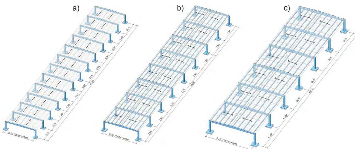
Übersicht der Hallenvarianten: a) Raster 5 m, b) Raster 7,5 m, c) Raster 10 m.
