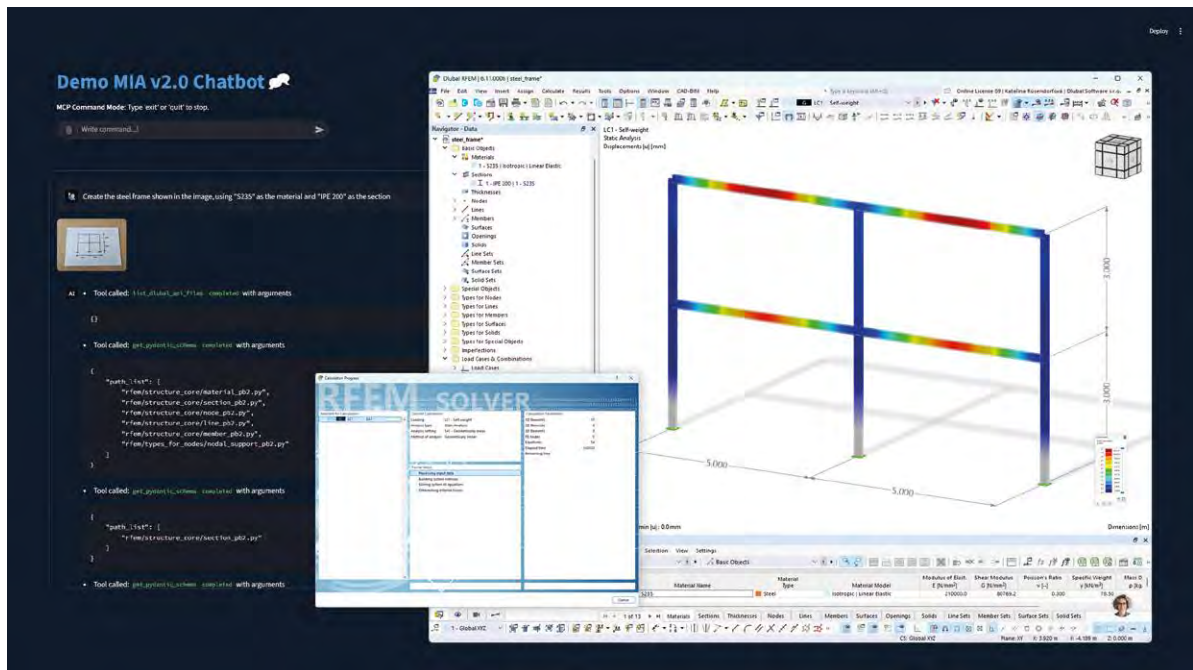
Demonstrator MIA: Aus einer Handskizze eines Kragarms (Material S235, Querschnitt IPE 200, drei Meter Spannweite) erstellt der KI-Agent selbstständig das Berechnungsmodell in der Finite-Elemente-Software.
