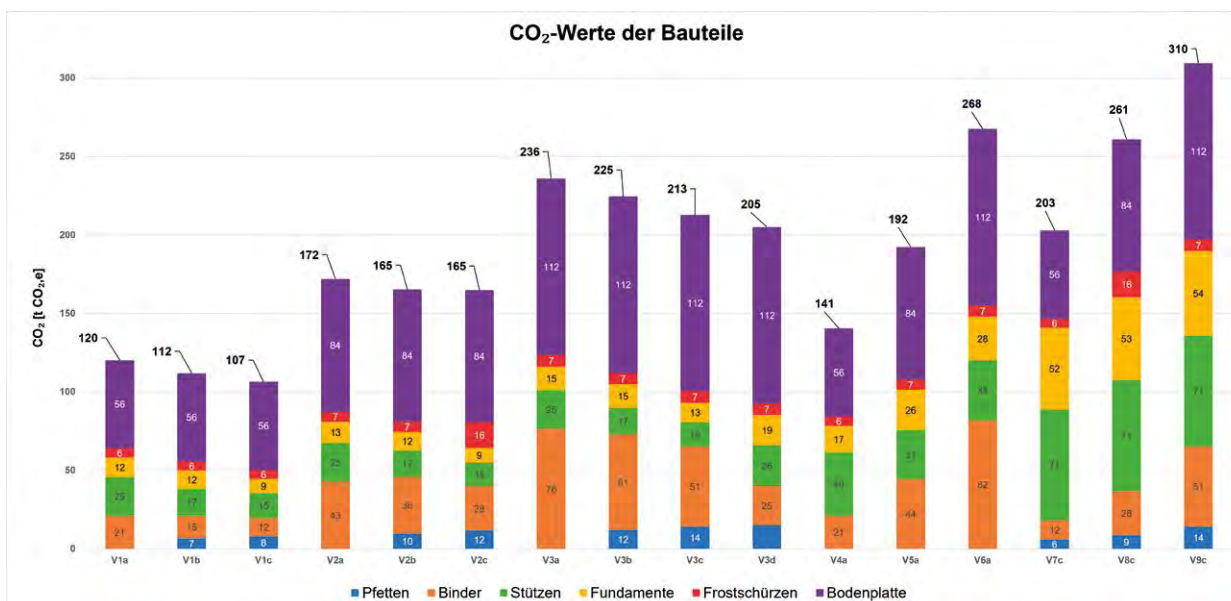
CO 2 -Werte der einzelnen Bauteile für die Hallenvarianten V1 bis V9.
