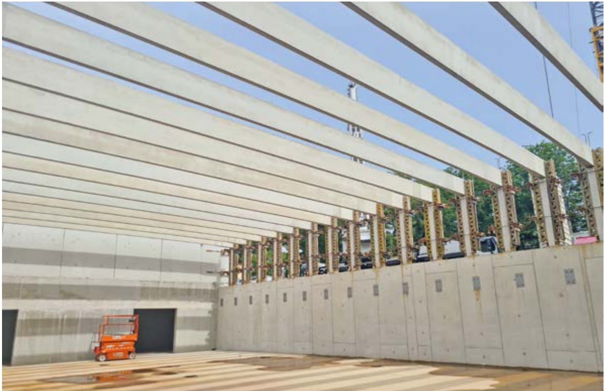
Turnhalle in Dresden: vorgespannte Carbonbetonbinder.
